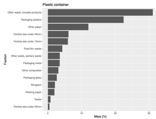
Fig. 6. Average raw material composition of plastic waste in a container Rys. 6. Średni skład surowcowy odpadów tworzyw sztucznych w pojemniku
