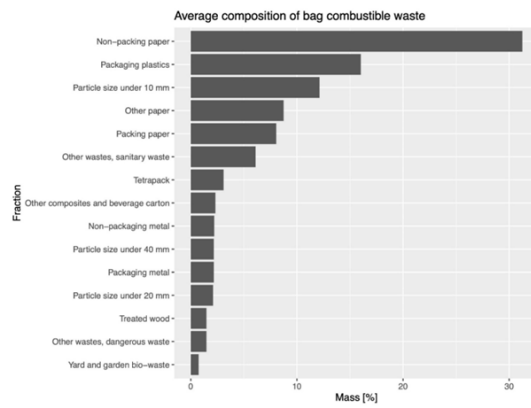
Fig. 5. Average raw material composition of combustible waste in bags Rys. 5. Średni skład surowcowy odpadów palnych w workach
